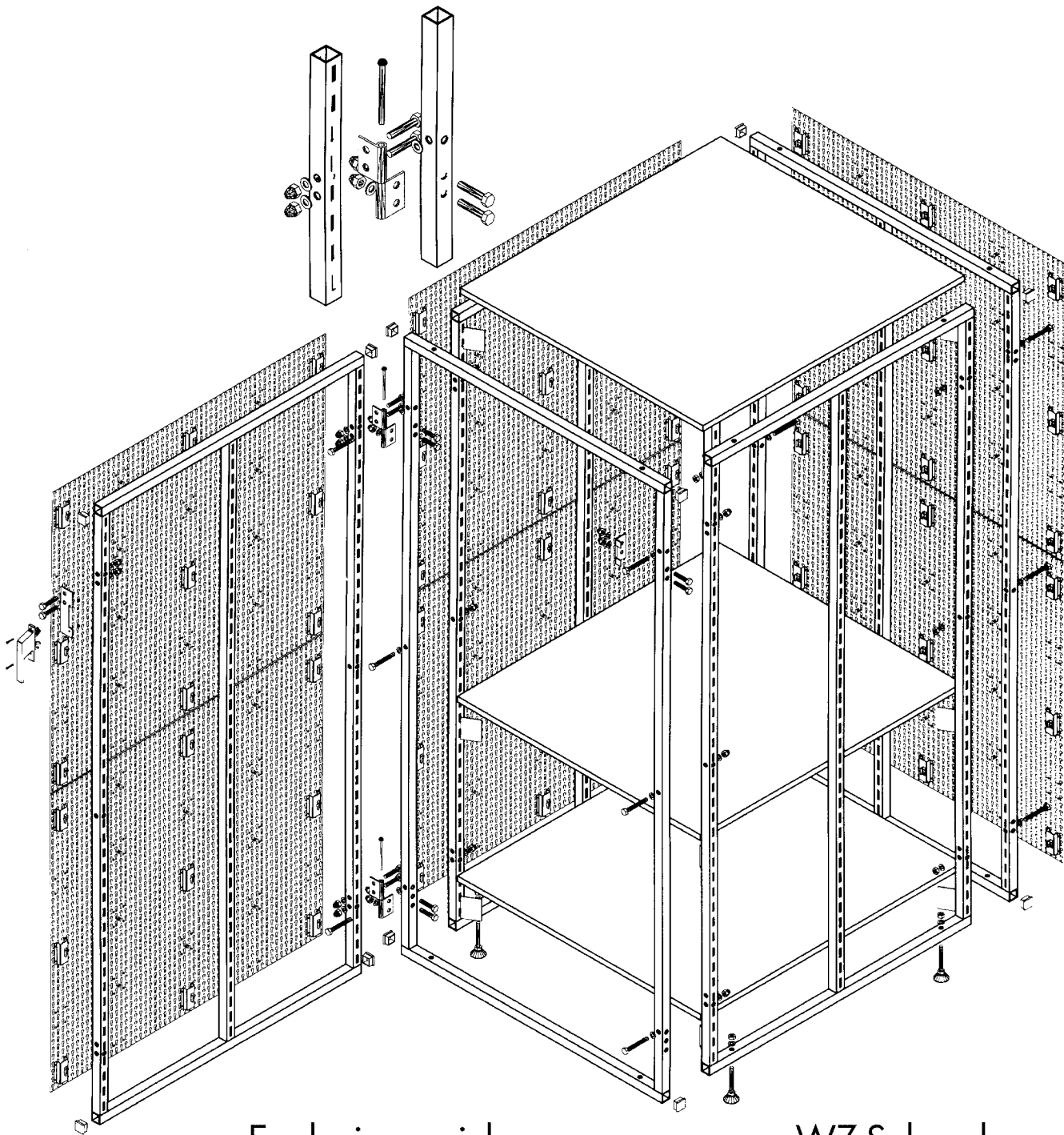
Explosionszeichnung
